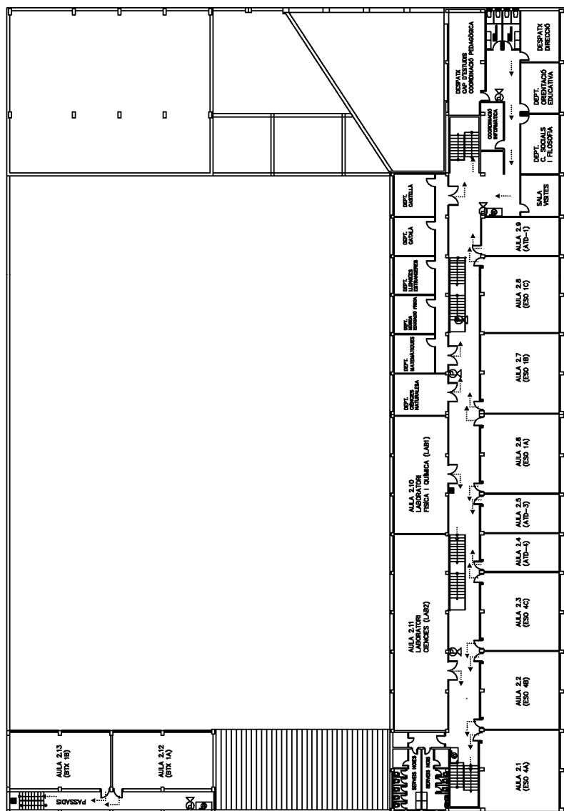
PLANTA 2 ESC: 1/250
